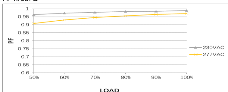
P.F vs LOAD
