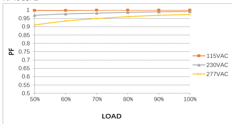
P.F vs LOAD
