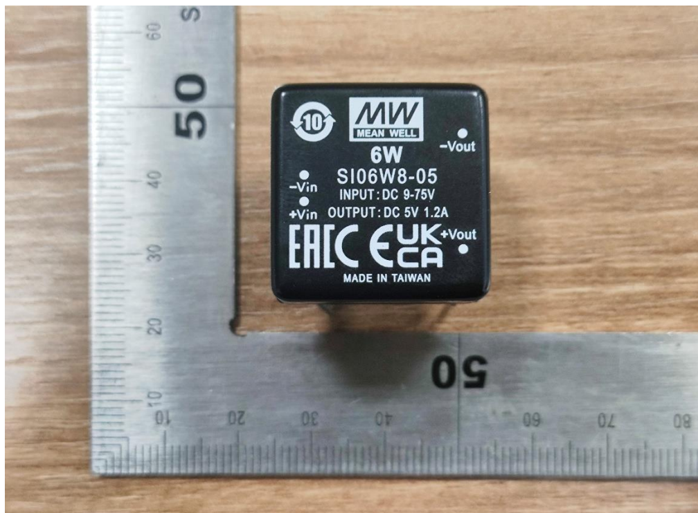
Bild / Picture 2: Overview
