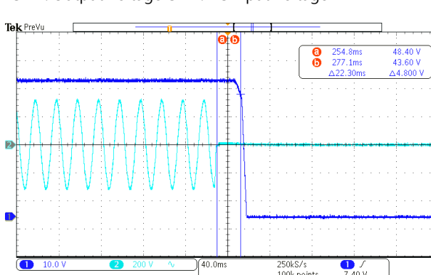
CH1 : Output Voltage CH2 : AC Input Voltage
