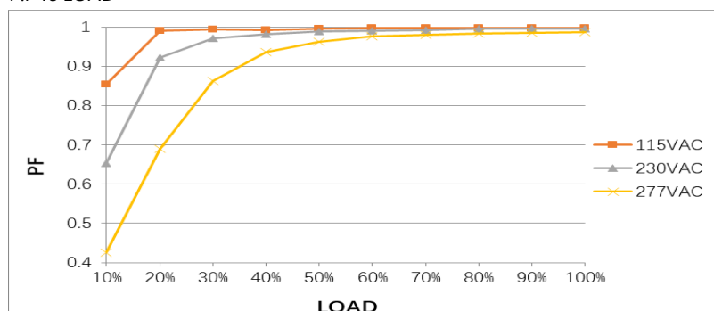
P.F vs LOAD
